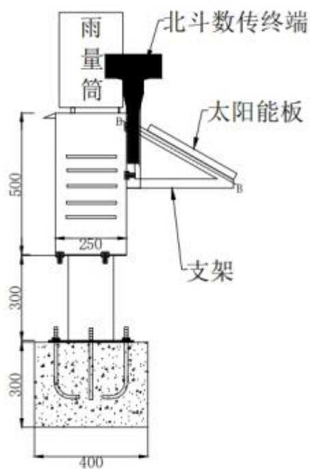
图 4.1-5 设备安装示意图
